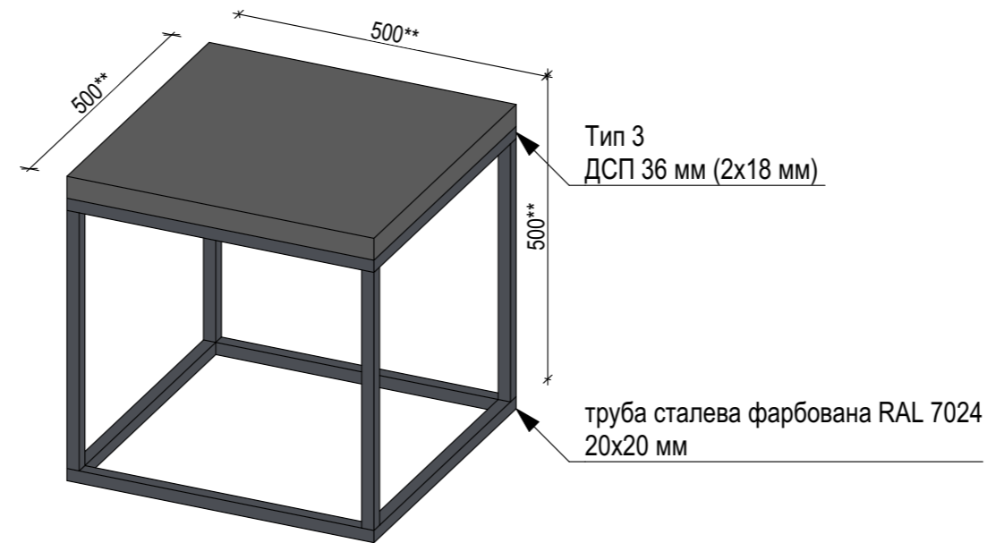
Аксометрія М-19
