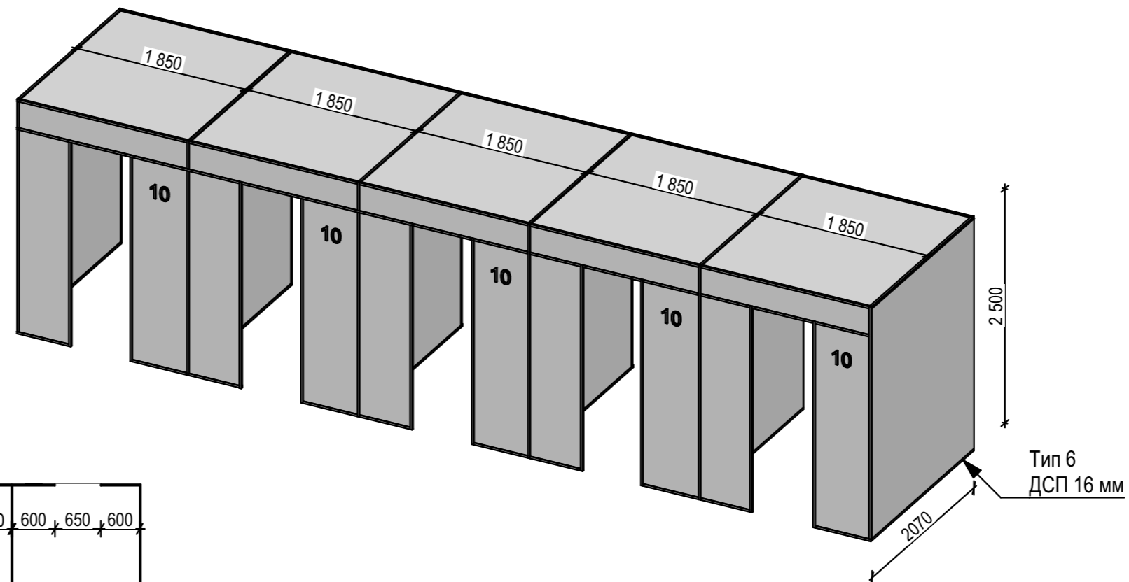
Аксонометрія
