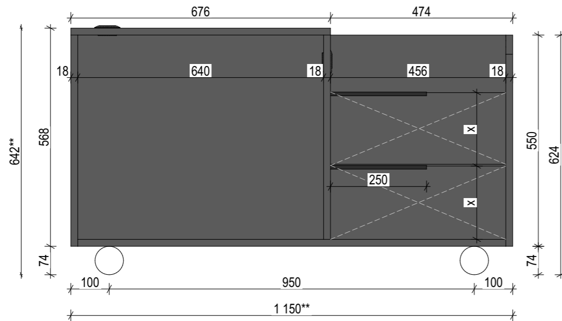
Вигляд спереду
