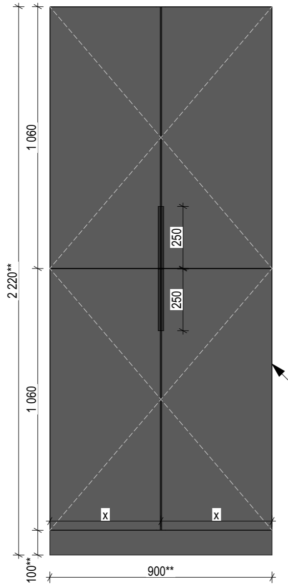
Вигляд спереду
