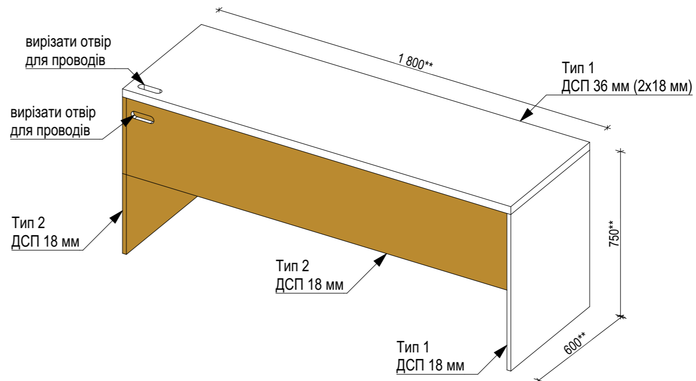
Аксонометрія
