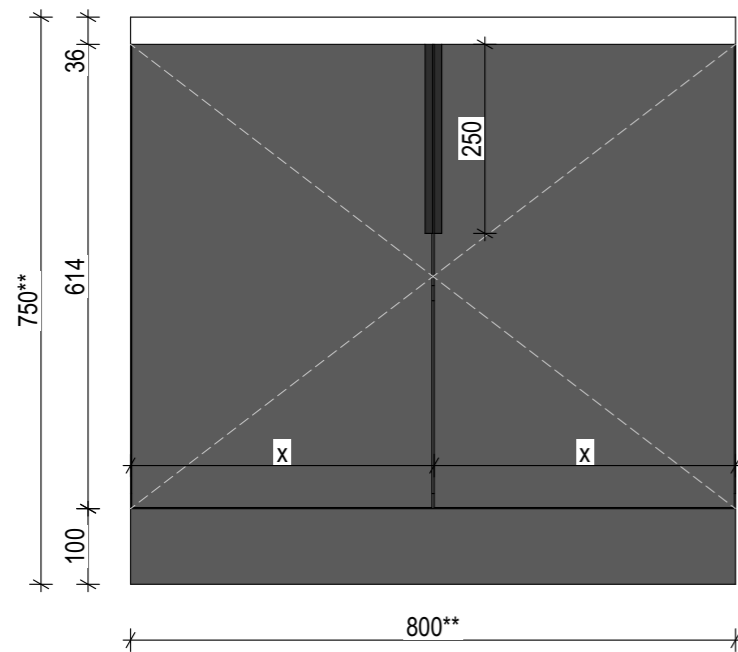
Вигляд спереду
