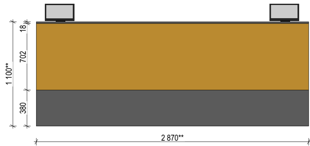
Вигляд спереду
