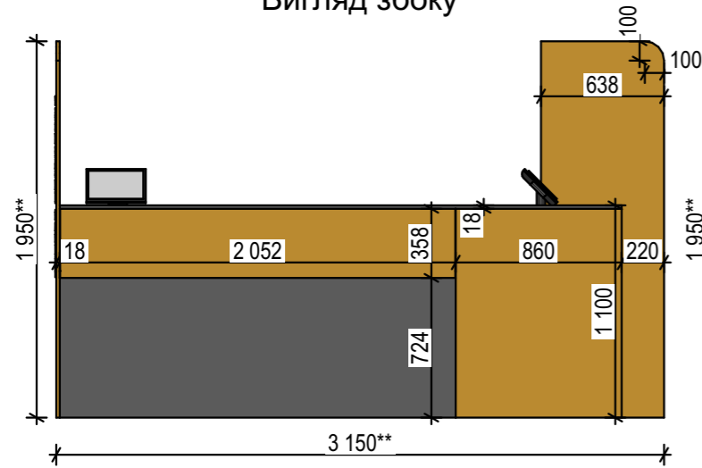
Вигляд збоку
