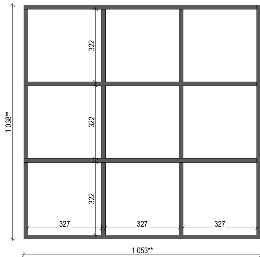
Вигляд спереду М-21
