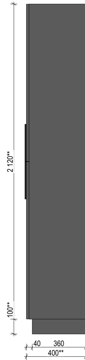
Вигляд збоку
