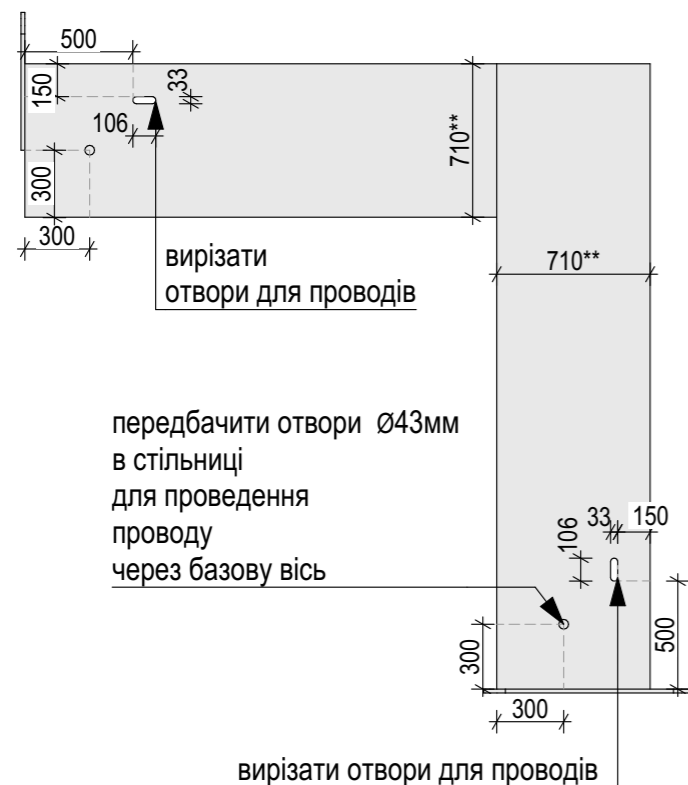
Вигляд згори на відмітці +750
