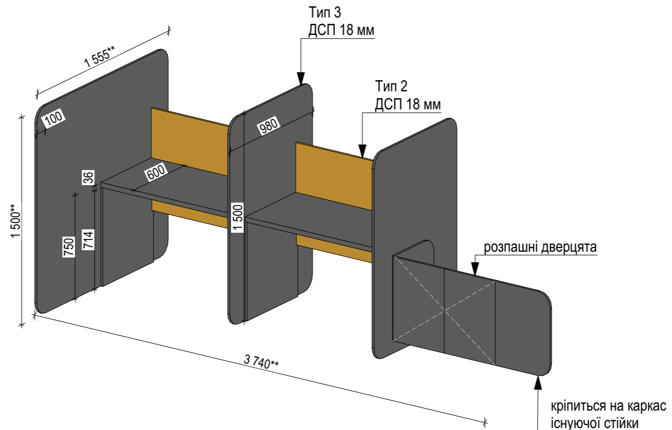
Аксонетрія
