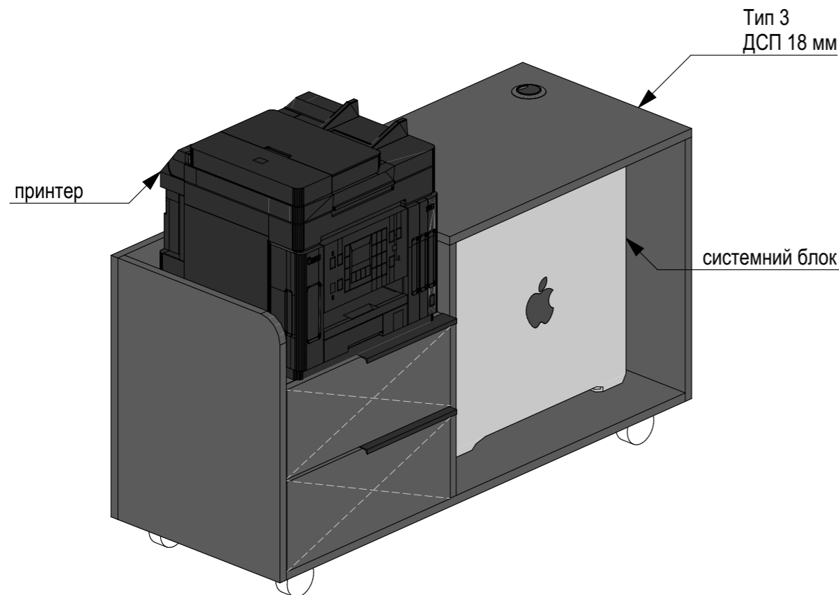
Аксонометрія
