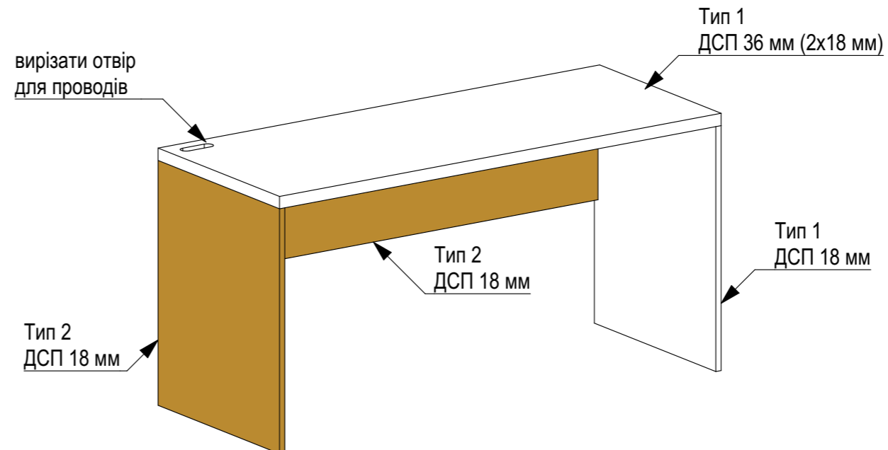
Аксометрія
