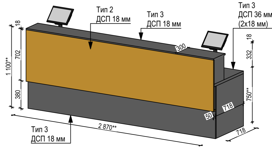
Аксонетрія
