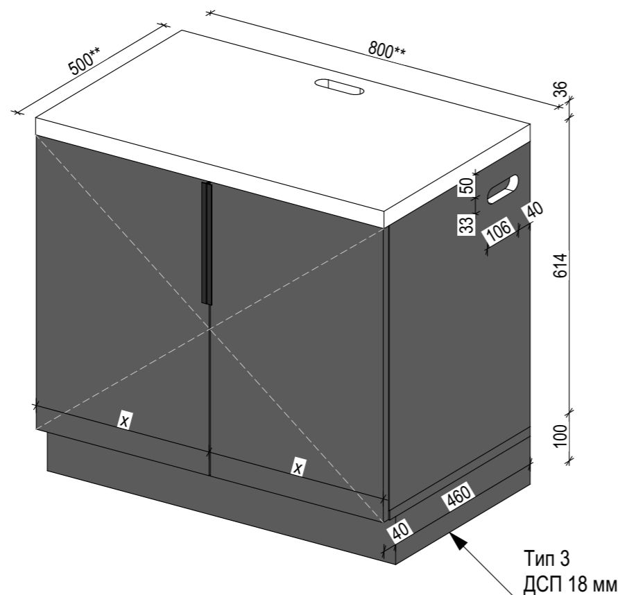
Аксонетрія
