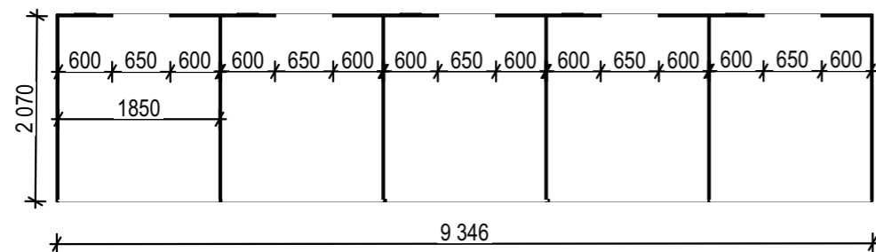
Вигляд згори
