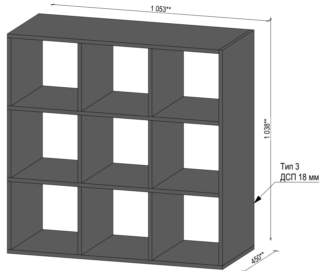
Аксометрія М-21
