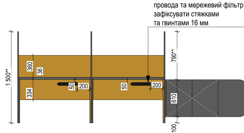
Вигляд ззаду
