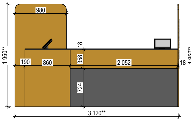
Вигляд збоку
