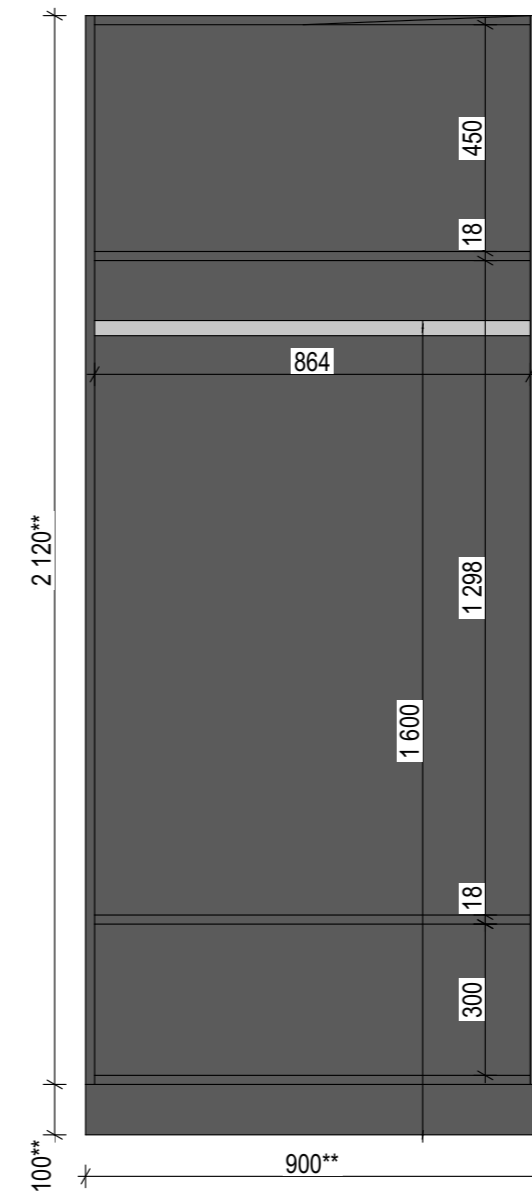
Внутрішнє наповнення
