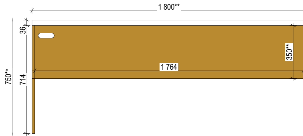
Вигляд спереду
