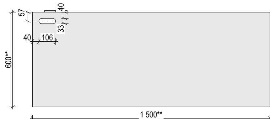
Вигляд згори
