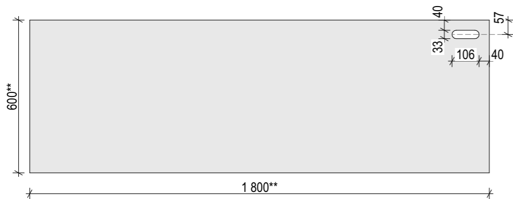
Вигляд згори
