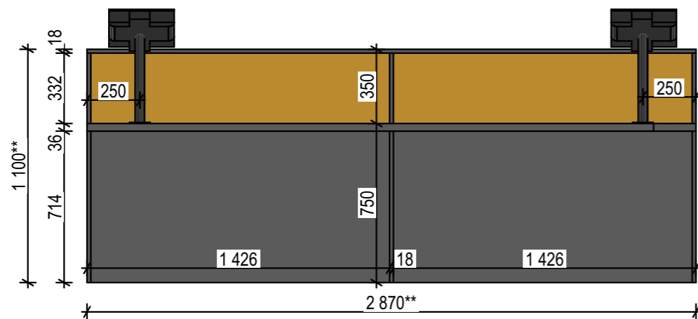
Вигляд ззаду
