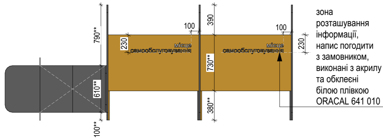
Вигляд спереду
