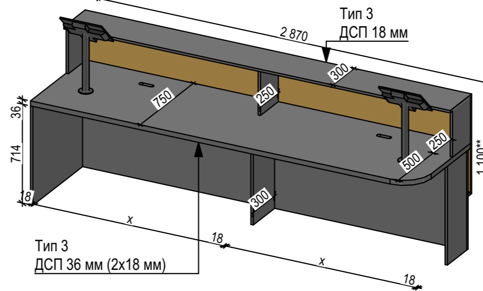
Аксонетрія
